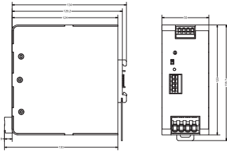
Maßzeichnung
